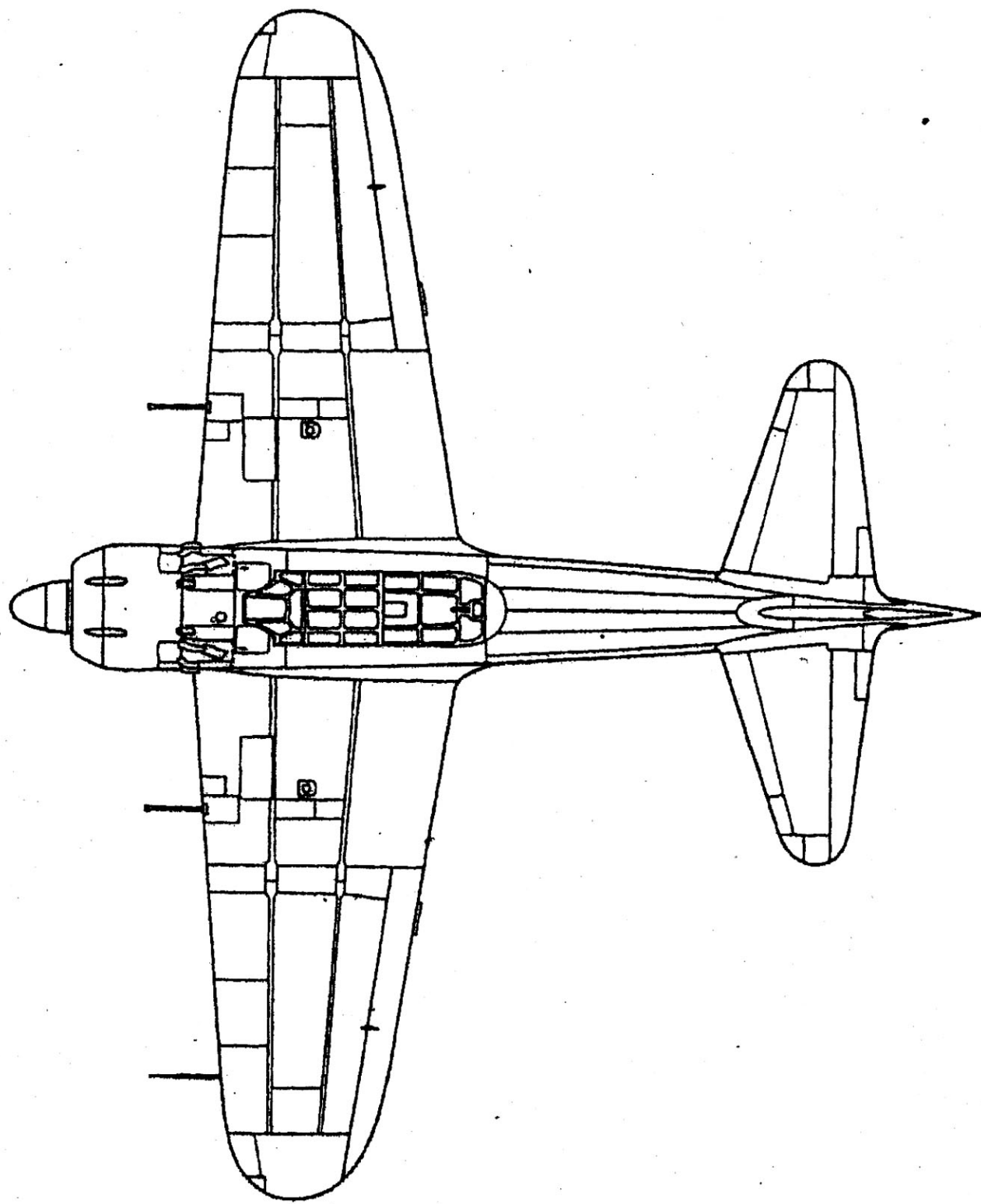
ゼロ式艦上戦闘機五二型 A6M5 (ゼロ戦)
